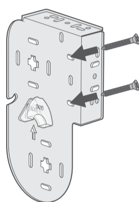
側面付け
