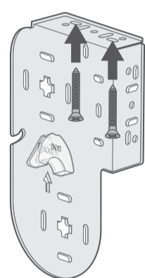
天井付け
