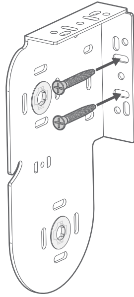
正面付け
